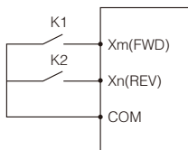
图 F7-3 二线式控制模式 2 示意图
