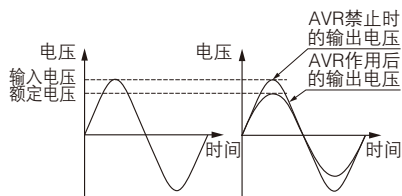
图 FC-2 AVR 功能示意图
