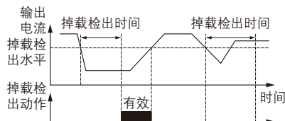
图 FA-3 掉载检出示意图
