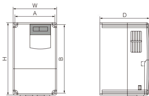
图A-1 7.5kW及以下机型的外形尺寸
