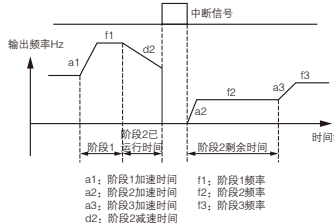
图 F9-4 PLC 启动方式 1
