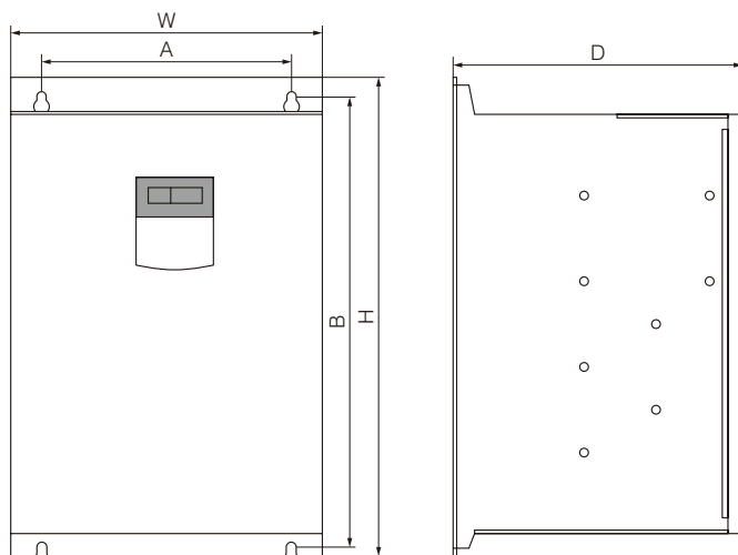
图A-2 22~132kW机型外形尺寸 (380V)
