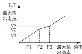
图 F5-2 用户设定 V/F 曲线示意图
