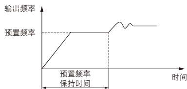
图 F8-4 闭环预置频率运行示意图
