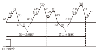
图 F9-3 PLC 连续循环示意图
