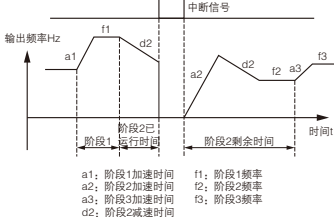
图 F9-5 PLC 启动方式 2
