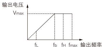
图 F0-1 电压与频率示意图
