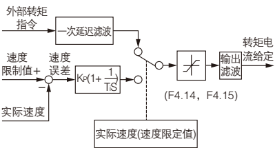
图 F4-2 转矩控制简化框图
