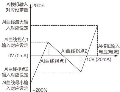
图 F6-2 多点曲线示意图
