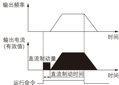
图 F1-2 启动直流制动示意图
