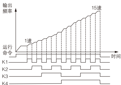
图 F7-1 多段速运行示意图
