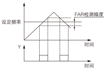
图 F7-7 频率到达示意图
