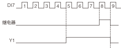
图 F7-9 计数器复位设定和计数器检测设定示意图
