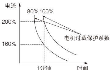
图 FA-1 电机过载保护曲线
