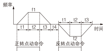
图 F1-5 点动运行图
