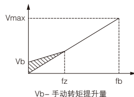
图 F5-3 转矩提升示意图
