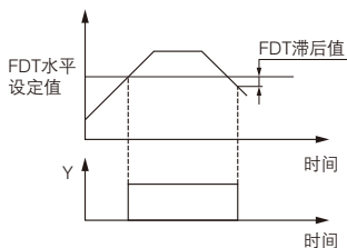
图 F7-8 频率水平检测示意图
