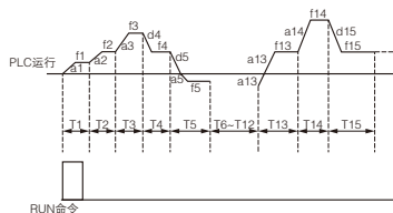
图 F9-2 PLC 单循环后保持示意图
