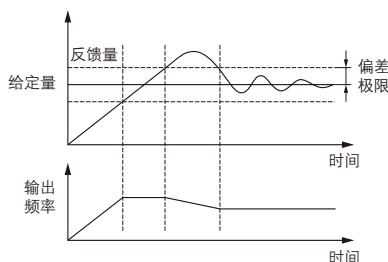
图 F8-3 偏差极限示意图
