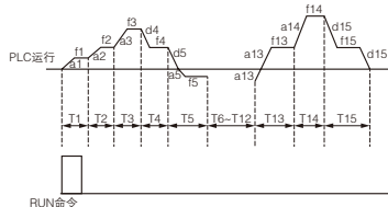
图 F9-1 PLC 单循环后停机示意图
