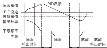
图 F8-5 第一种睡眠模式示意图
