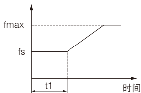
图 F1-1 启动频率示意图
