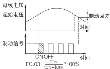
图 FC-1 能耗制动示意图
