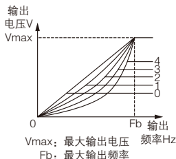
图 F5-1 V/F 曲线示意图
