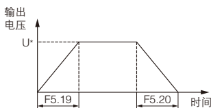
图 F5-7 电压控制模式 2
