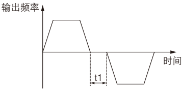
图 F1-7 正反转死区时间示意图
