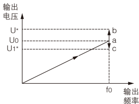
图 F5-4 电压控制模式 0
