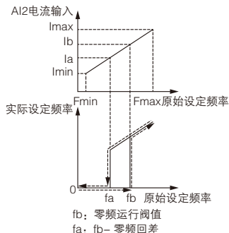
图 F6-1 零频功能示意图
