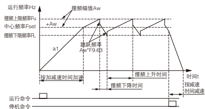
图 F9-6 摆频示意图
