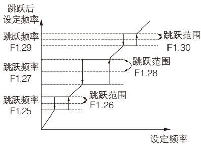
图 F1-6 跳跃频率示意图
