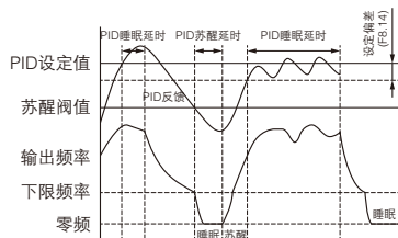
图 F8-6 第二种睡眠模式示意图
