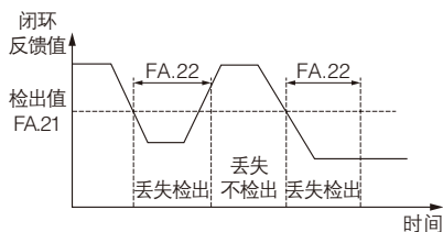
图 FA-4 闭环反馈丢失检出时序图
