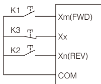
图 F7-4 三线式控制模式 1 示意图
