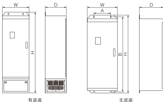
图A-3 160~350kW机型外形尺寸 (380V)
