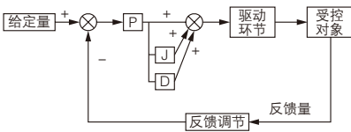
图 F8-2 PID 调节示意图
