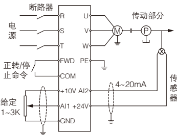
图 F8-1 模拟反馈控制系统示意图
