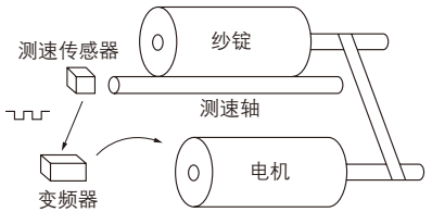
图 F9-7 长停机功能举例图
