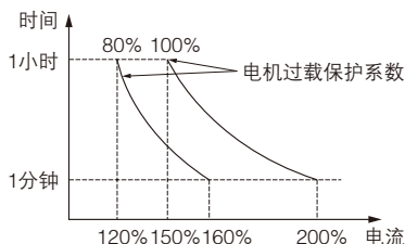
图 FA-2 电机过载保护系数设定示意图
