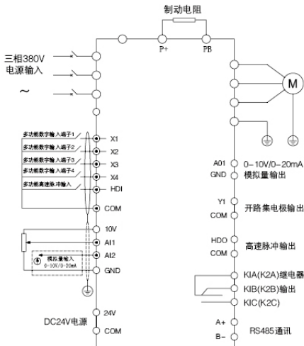
图 2-2 变频器控制回路接线方式
