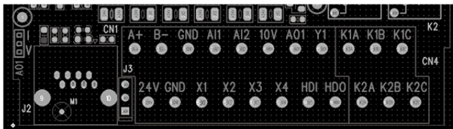
图 2-3 70（非隔离版本）控制回路端子布置图
