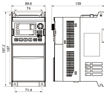
70 系列 0.75-2.2KW 外形及安装尺寸图
