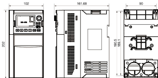
70 系列 3-7.5KW 外形及安装尺寸图
