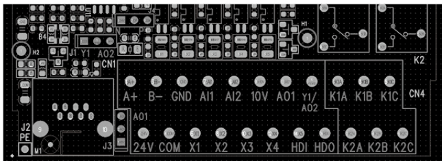
图 2-4 70（隔离版本）控制回路端子布置图
